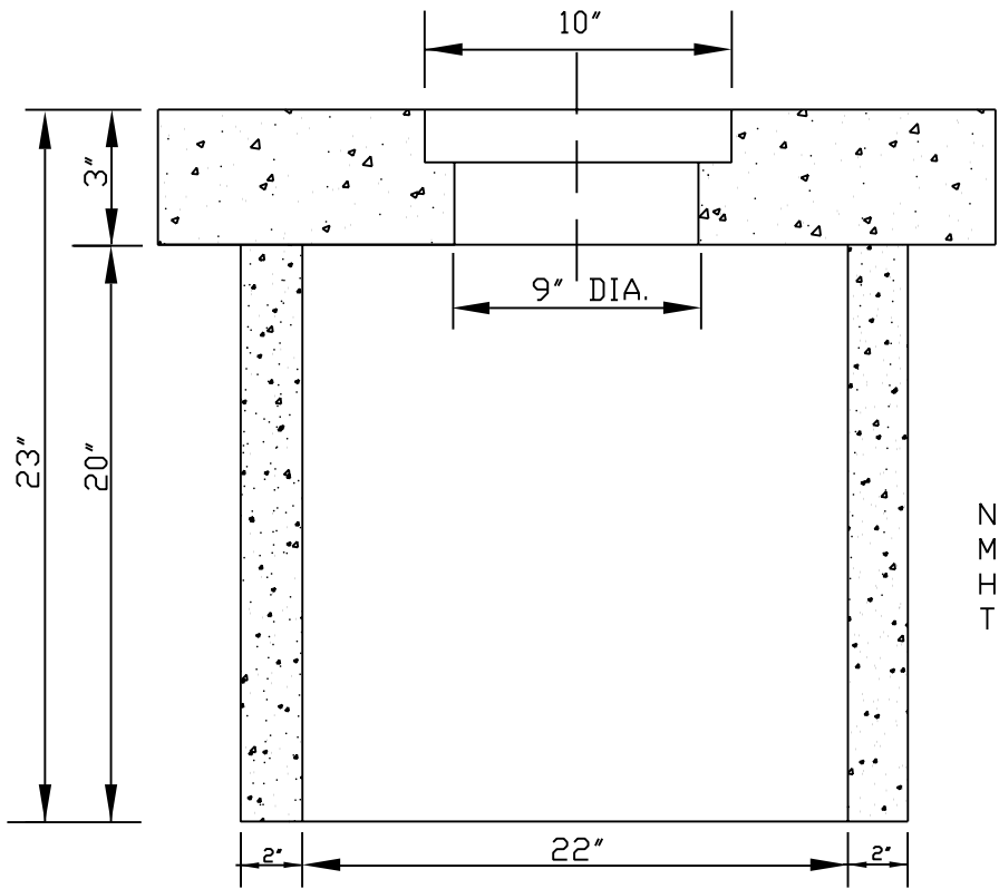
ELEVATION
