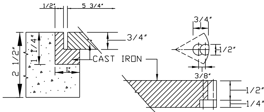
SECTION THRU RING LID
